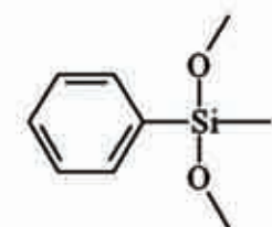
Dimethoxymethylphenylsilane
